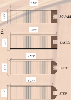
STANDARD EDGE DETAIL
